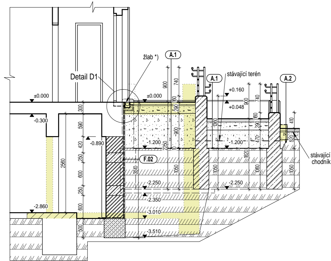
Řez C-C
