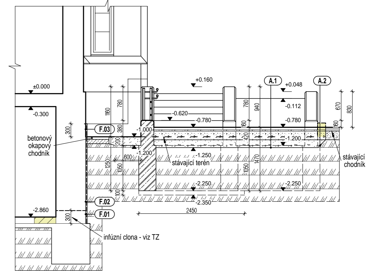
Řez D-D
