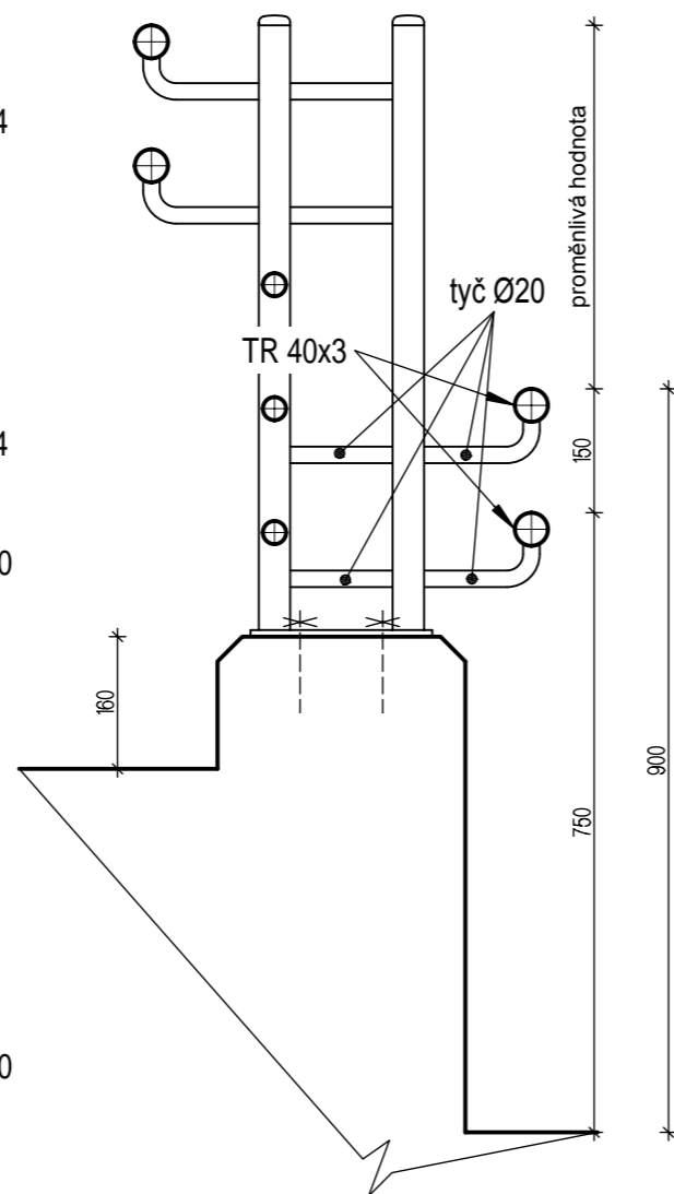
Detail D5 - M 1:10
